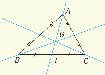
G es baricentro y punto de intersección de las transversales de gravedad.
